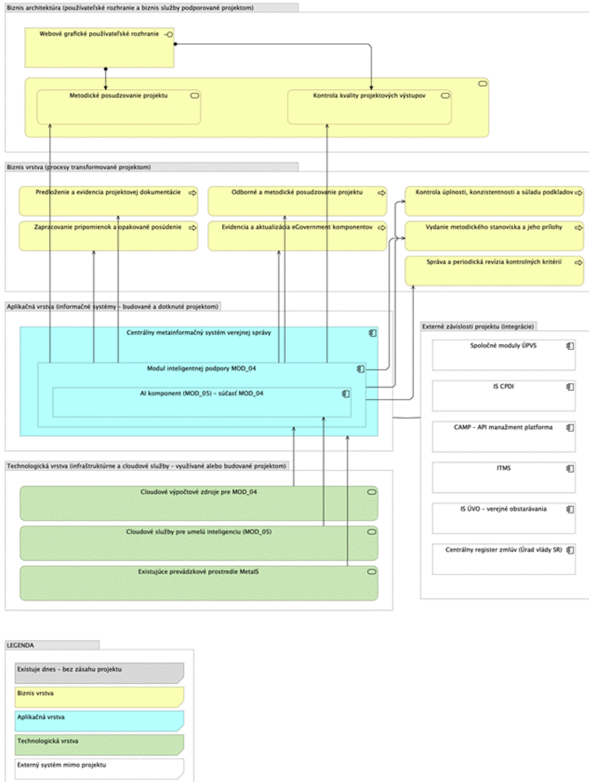
Obrázok 4 – Prehľad architektúry riešenia MetaIS+
