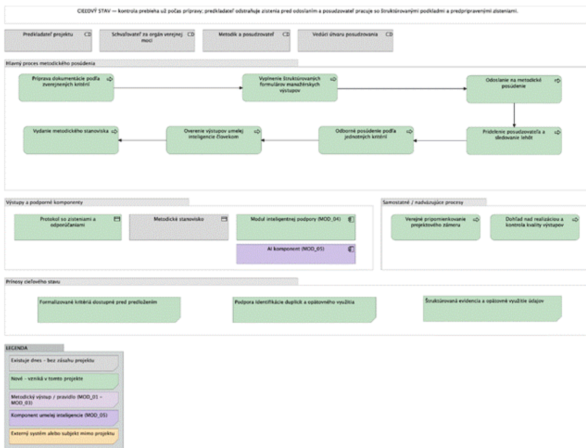
Obrázok 8 – Biznis vrstva – cieľový stav (TO BE)
